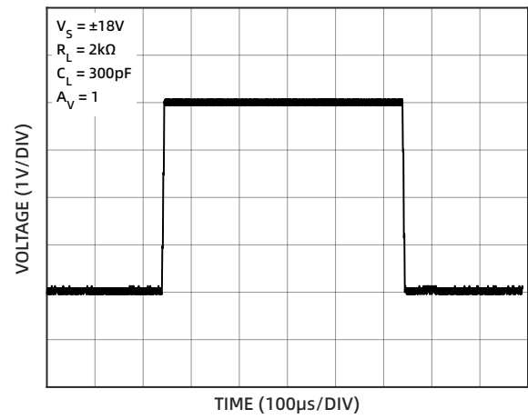
图 8 大信号瞬态响应 ( \pm 18V )
