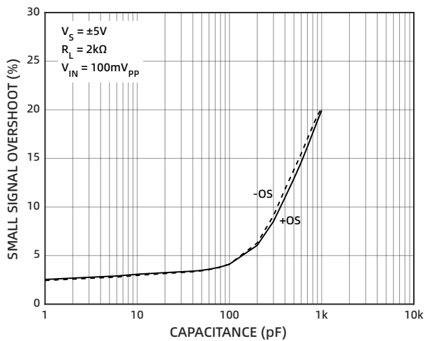
图 11 小信号过冲与负载电容的关系 ( \pm 5V )
