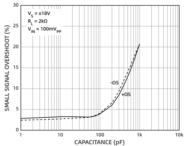
图 12 小信号过冲与负载电容的关系 ( \pm 18V )
