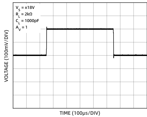
图 10 小信号瞬态响应 ( \pm 18V )
