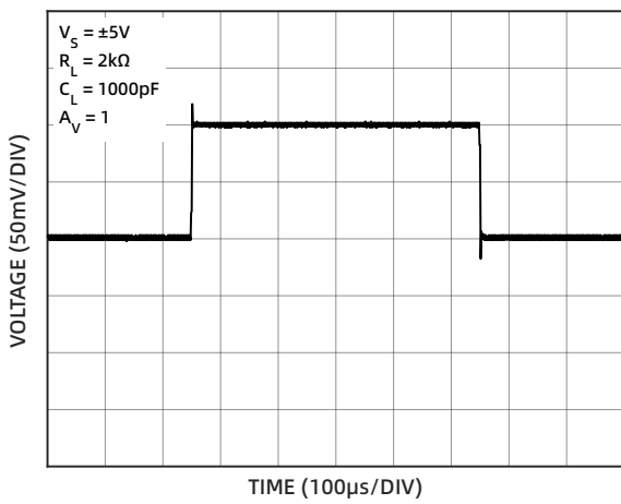
图 9 小信号瞬态响应 ( \pm 5V )
