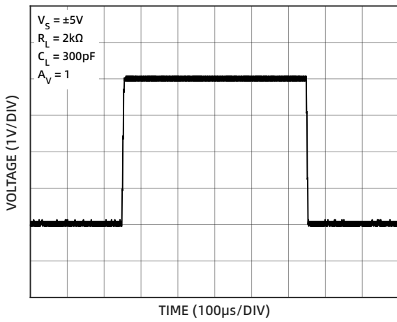
图 7 大信号瞬态响应 ( \pm 5V )
