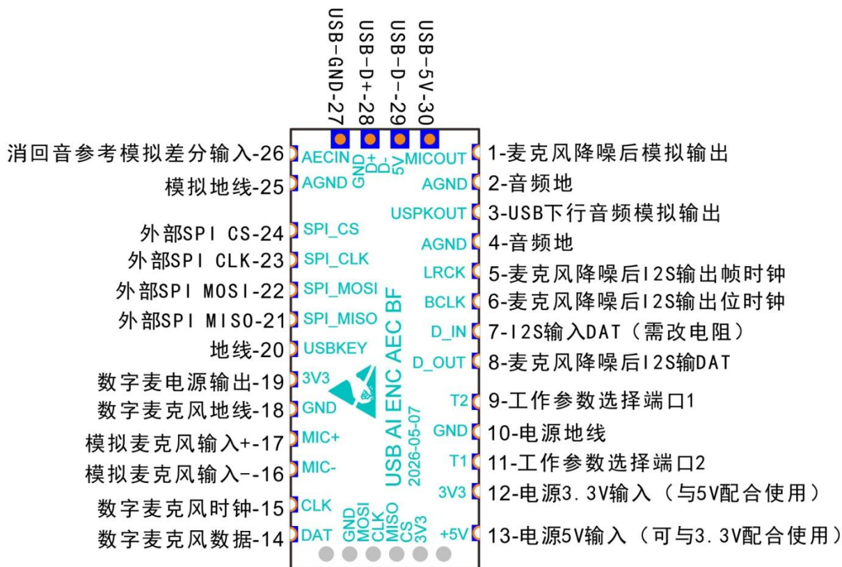
模块外形及功能端口示意图 正面（TOP）
