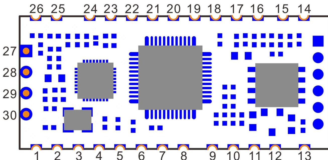
模块外形及功能端口示意图 正面（TOP）
