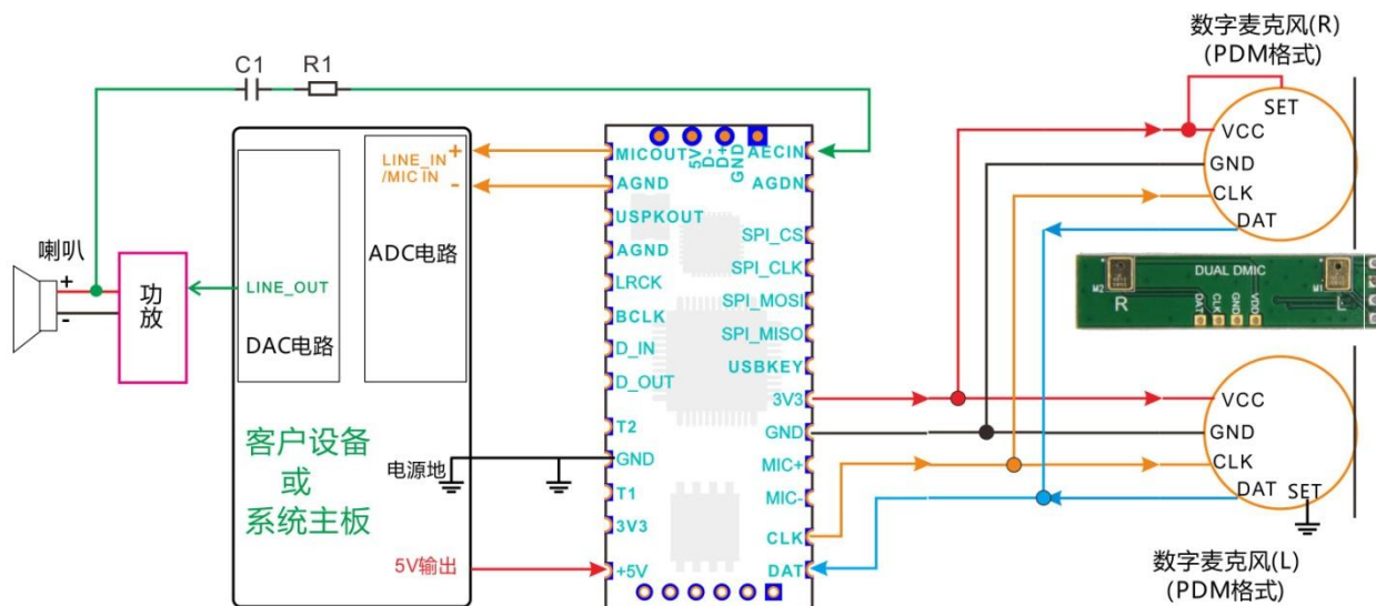
双数字麦克风+定向波束定向拾音+AI 降噪通话模拟连接（模式八）
