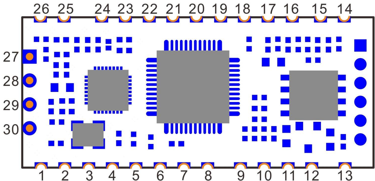
模块外形及功能端口示意图 正面（TOP）
