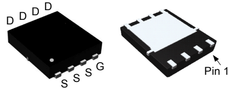
PDFN5*6-8L
