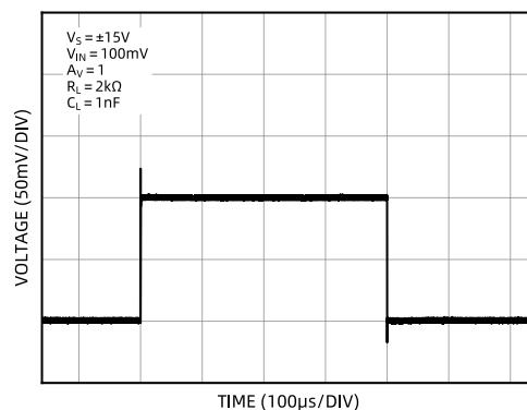
图 42 驱动容性负载
