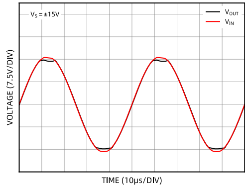
图 38 输出反相
