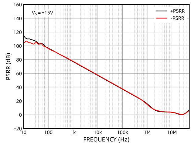
图 34 PSRR
