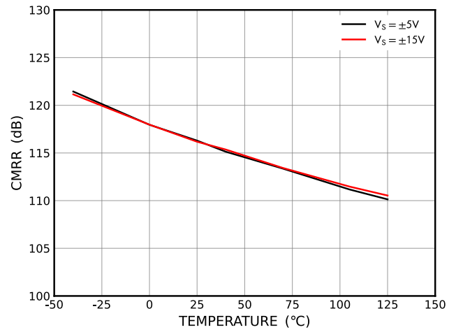
图 32 CMRR
