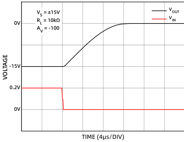
图 31 负向过载恢复
