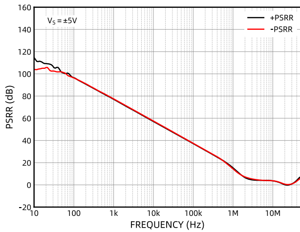
图 33 PSRR
