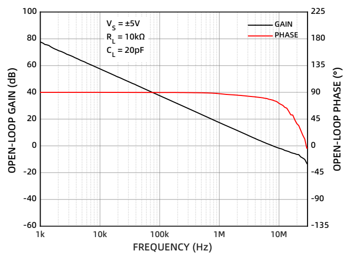
图 18 开环增益
