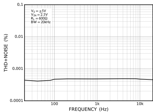
图 39 总谐波失真和噪声
