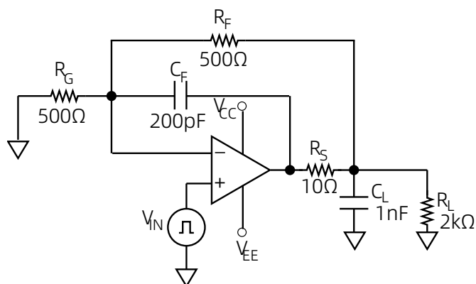
图 43 推荐容性负载电路
