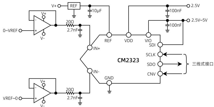
图 28 采用多个电源的典型应用电路
