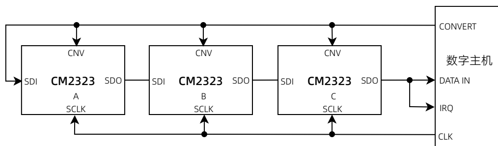
图 27 有繁忙指示连接图（级联模式）
