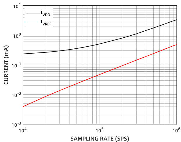
图 14 电流随采样率的变化
