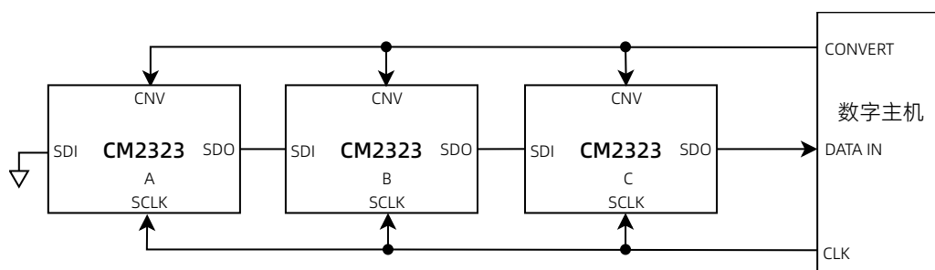
图 26 无繁忙指示连接图（级联模式）
