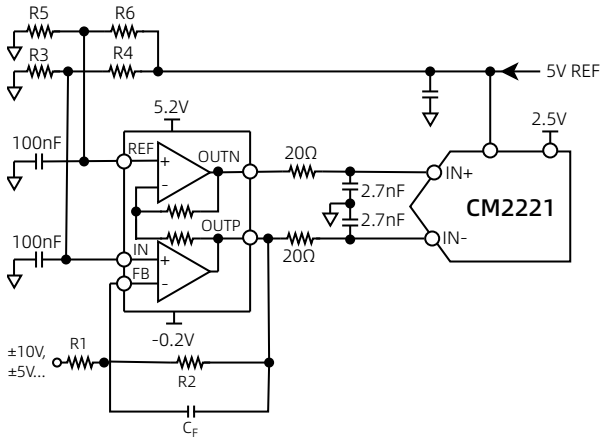
图 20 单端转差分驱动器电路
