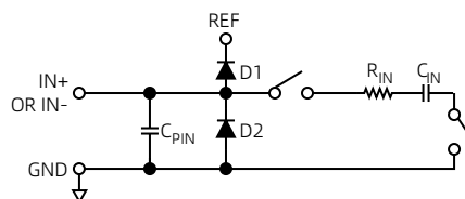
图 17 等效模拟输入电路
