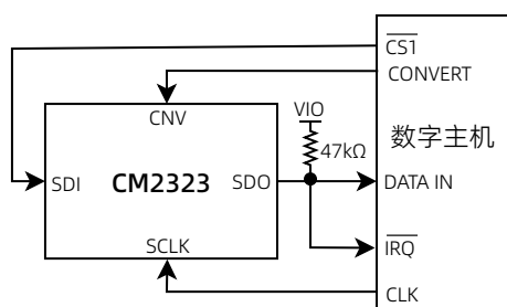
图 25 四线串口有繁忙指示连接图（片选模式）
