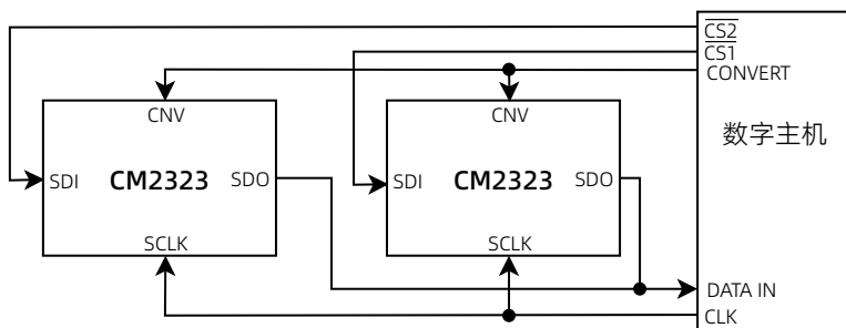
图 24 四线串口无繁忙指示连接图（片选模式）
