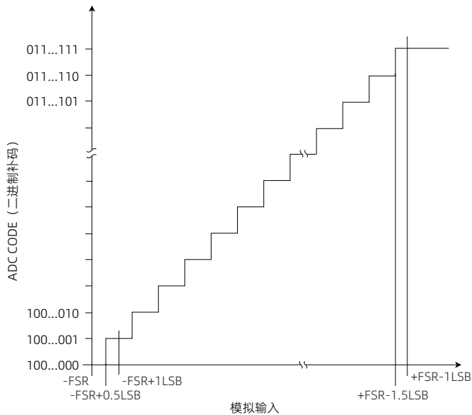
图 19 传递特性
