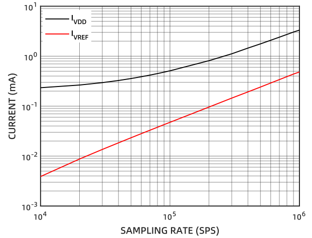
图 21 工作电流随采样率的变化
