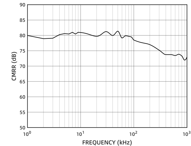
图 18 模拟输入 CMRR
