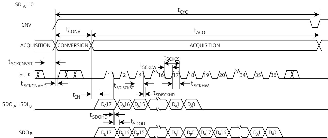
图 5 无繁忙指示串行接口时序（级联模式）
