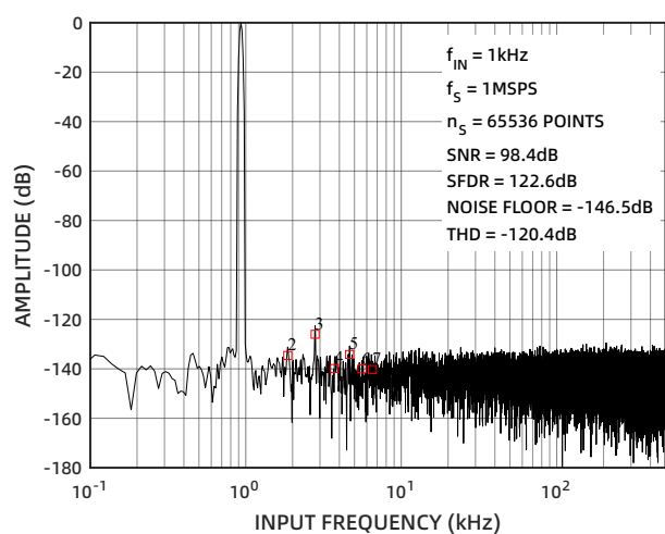
图 15 FFT, VREF = 5V
