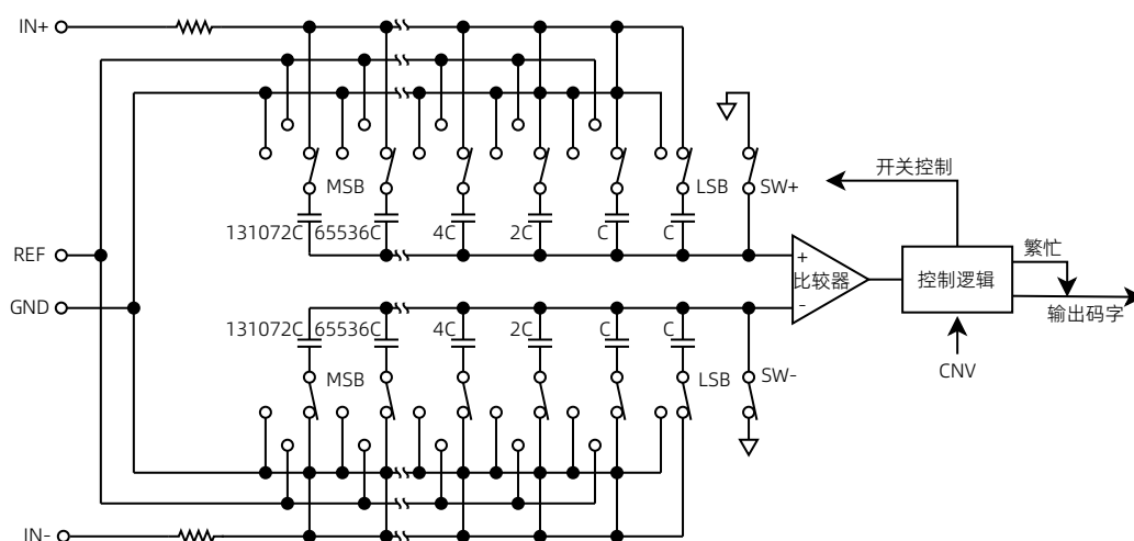
图 16 ADC 原理示意图
