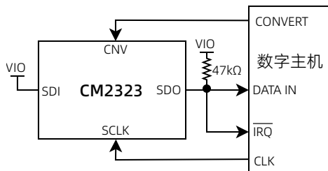
图 23 三线串口有繁忙指示连接图（片选模式）
