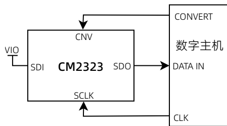
图 22 三线串口无繁忙指示连接图（片选模式）
