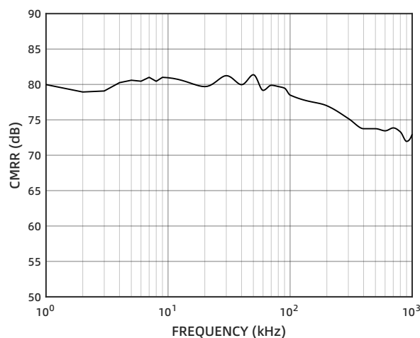
图 18 模拟输入 CMRR
