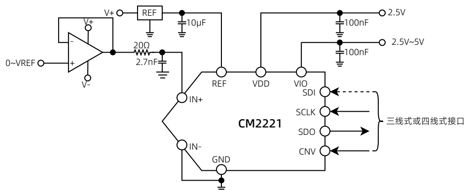
图 28 采用多个电源的典型应用电路
