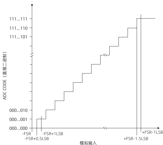
图 19 传递特性
