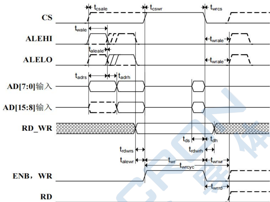
图 8-16: 复用寻址写周期时序
