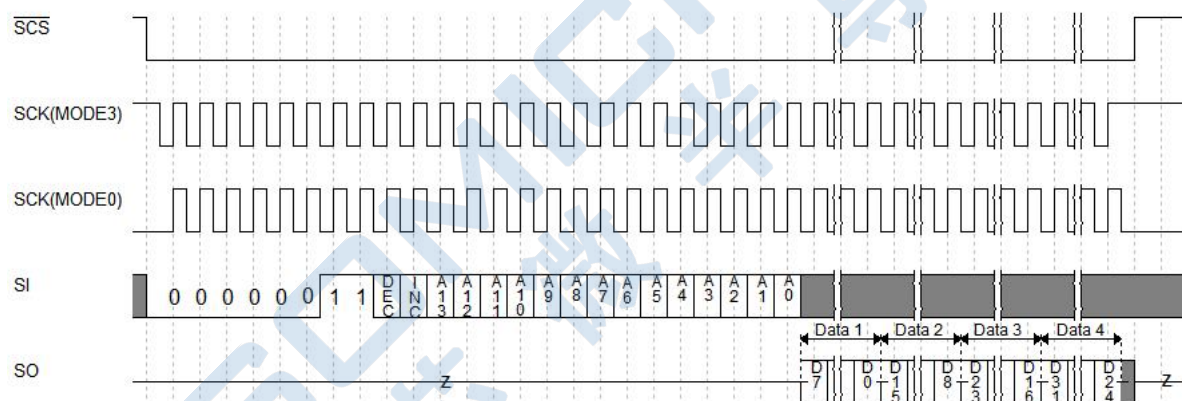
图 9 - 4: SPI 读取
