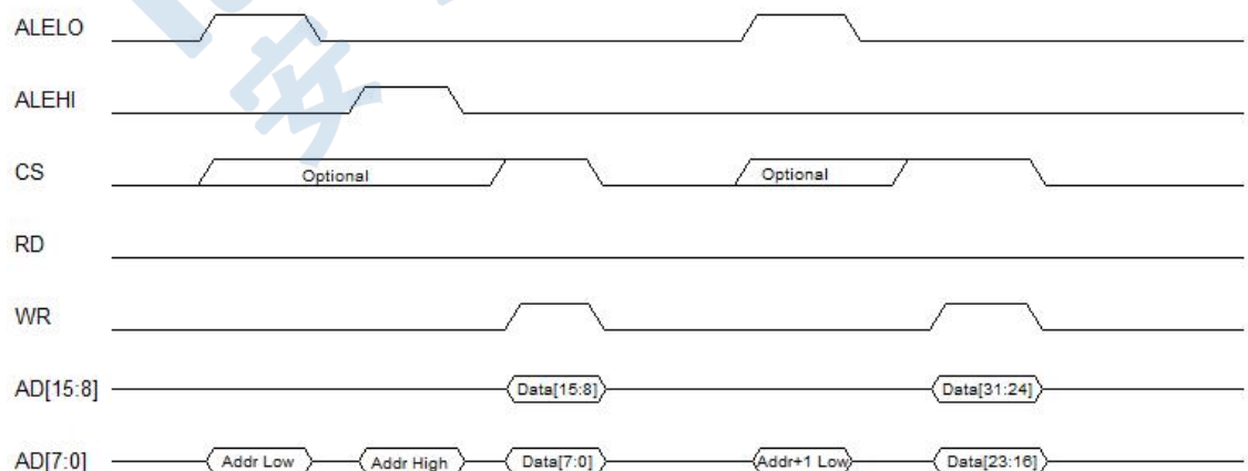
图 8-4：采用双相锁存的复用寻址 - 无 ALEHI 的 16 Bit 写
