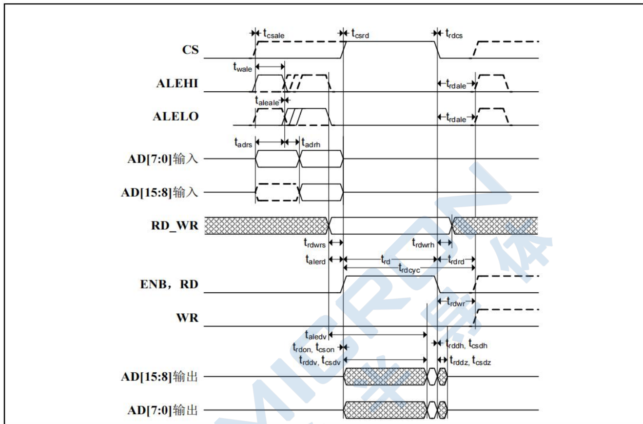
图 8-15: 复用寻址读周期时序
