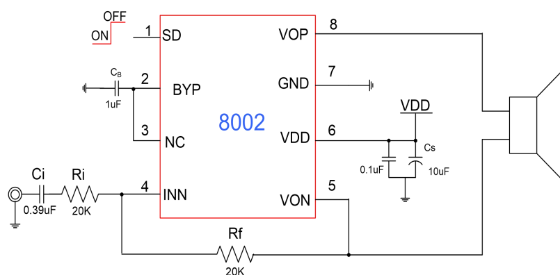
图1 WD8002D典型应用电路
