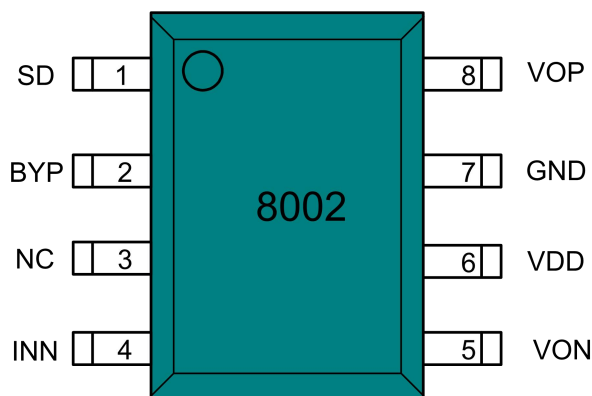
图2 WD8002D管脚定义
