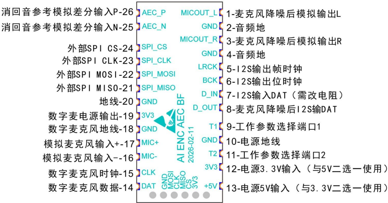
模块外形及功能端口示意图 背面（BOTTOM）
