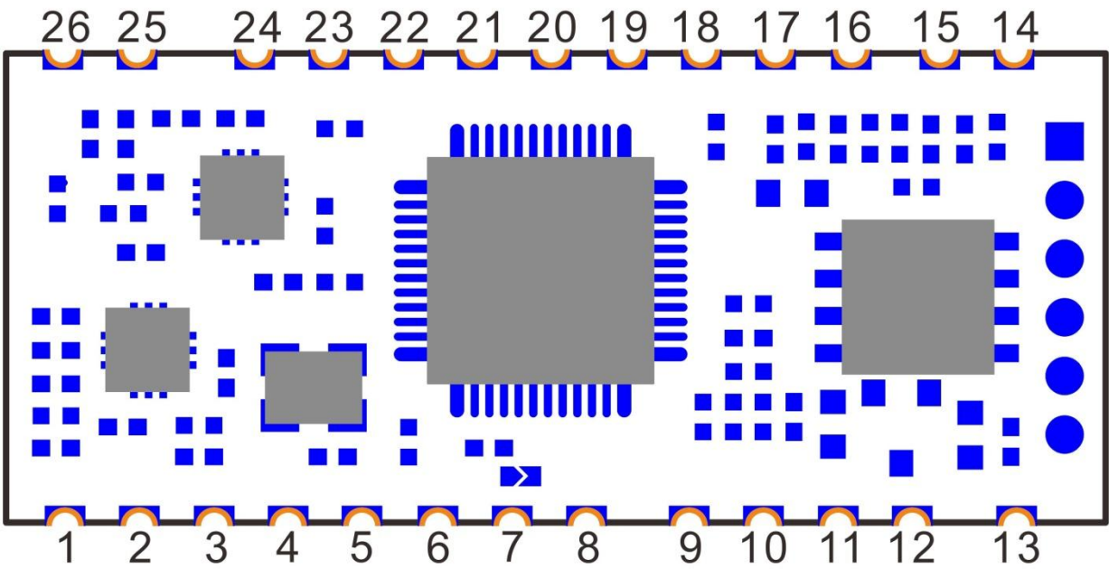
模块外形及功能端口示意图 正面（TOP）
