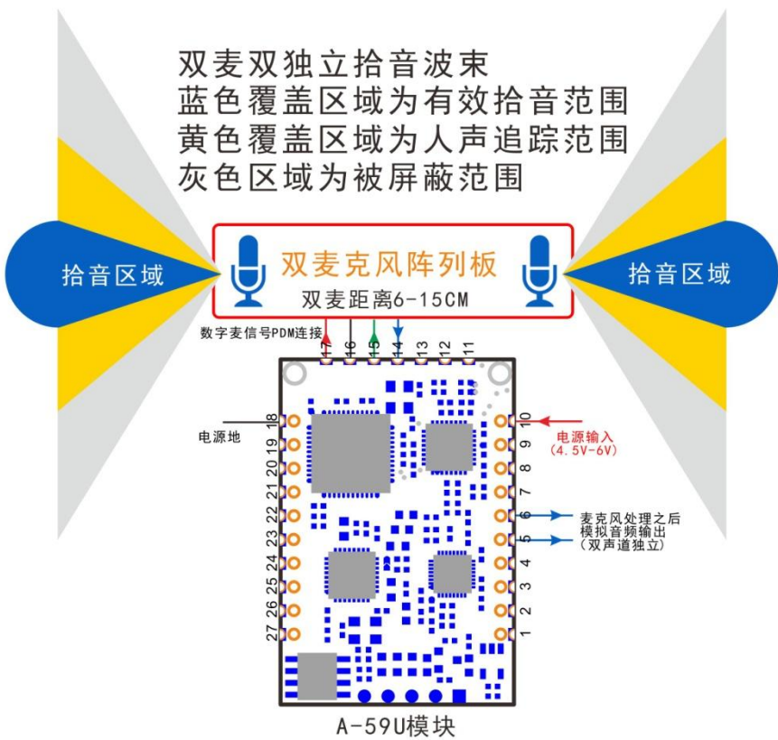
A-59U 模块配合双麦克风的双拾音波束示意图
