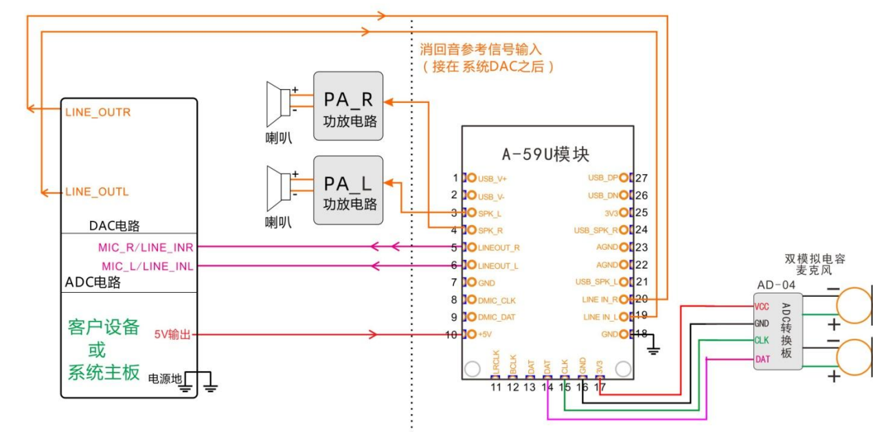
模拟麦克风输入功放接在模组之后（消回音模式六）
