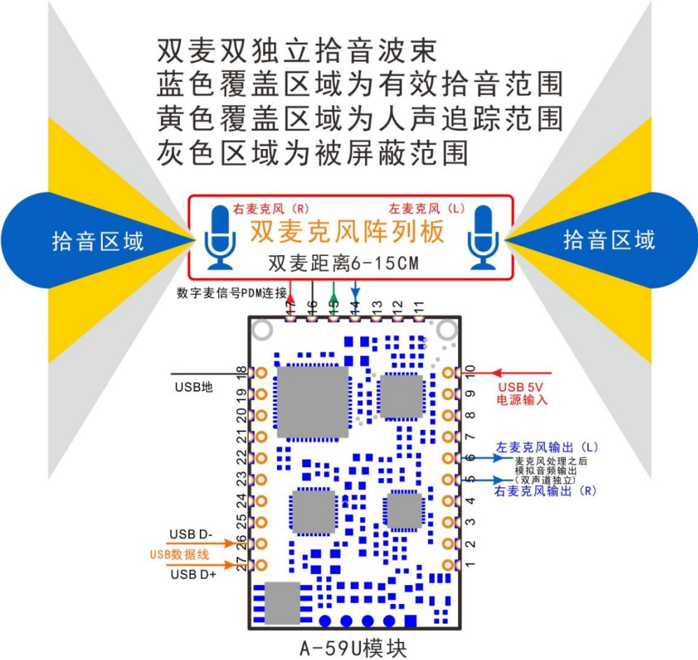
A-59U 模块 USB 数据线连接方式
