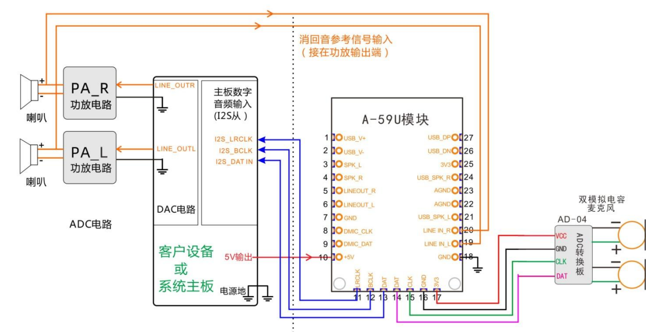
模拟麦克风输入数字音频输出（消回音模式七）
