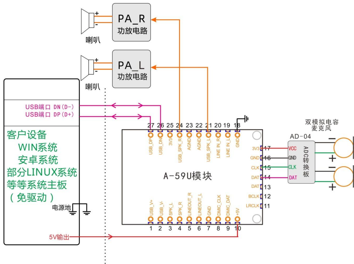
USB 系统连接 双模拟电容麦克风模式（消回音模式十）
