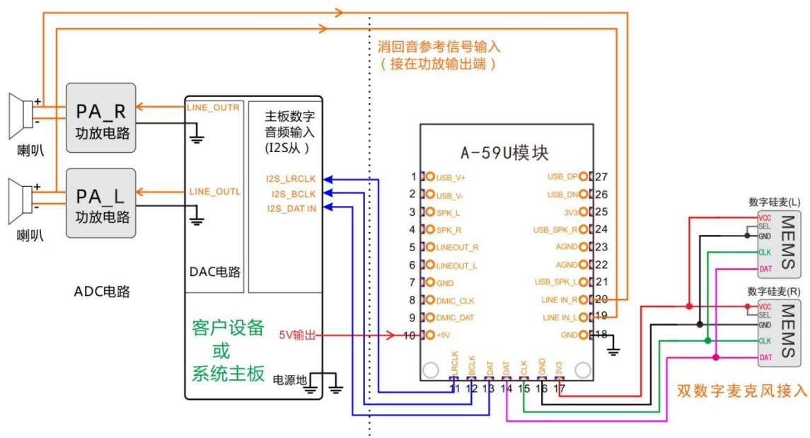
数字音频输出连接模式（消回音模式三）
