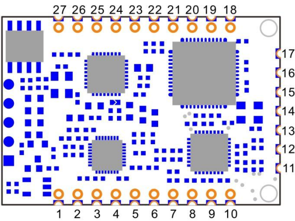
模块外形及接口示意图
