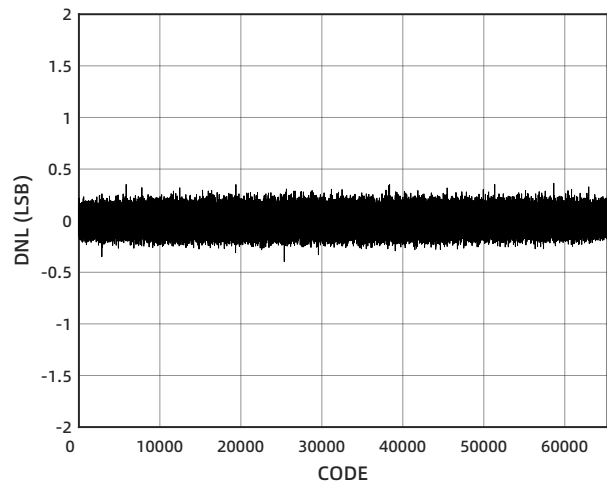
图 10 DNL
