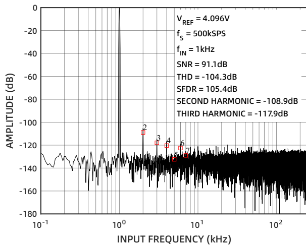
图 19 FFT (4V)
