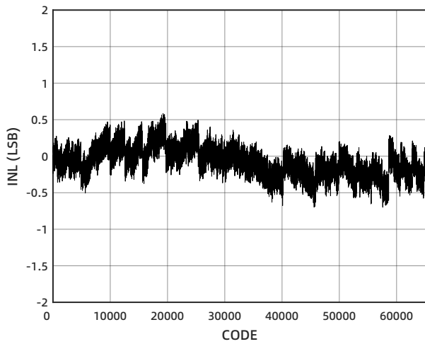
图 9 INL
