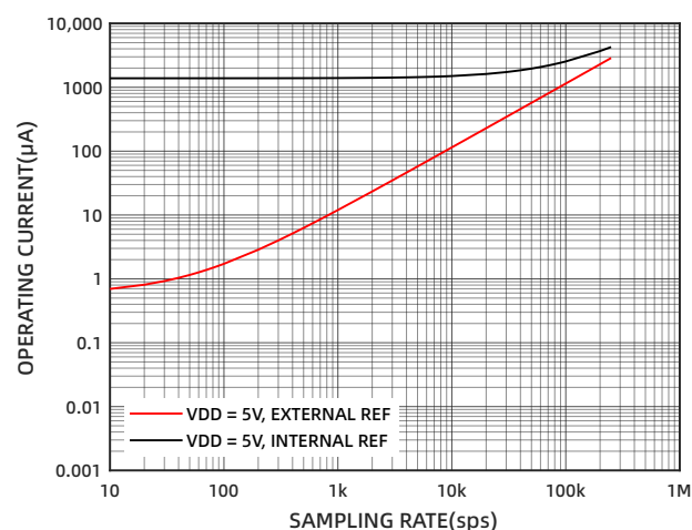
图 24 工作电流与采样率的关系
