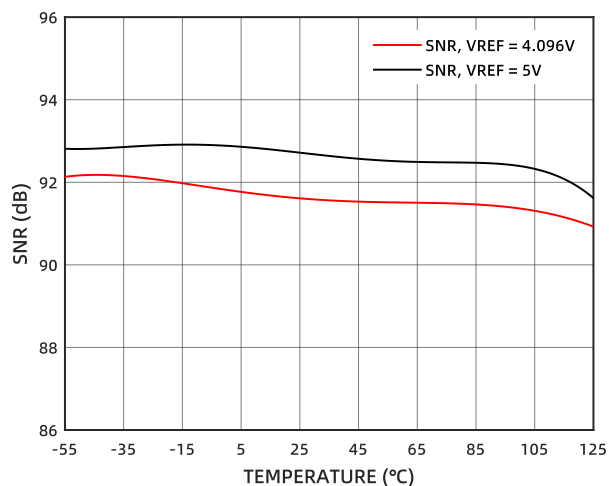
图 13 SNR 的温度特性
