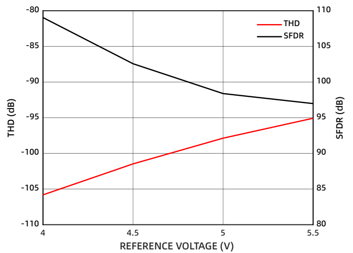
图 12 THD、SFDR 与基准电压的关系
