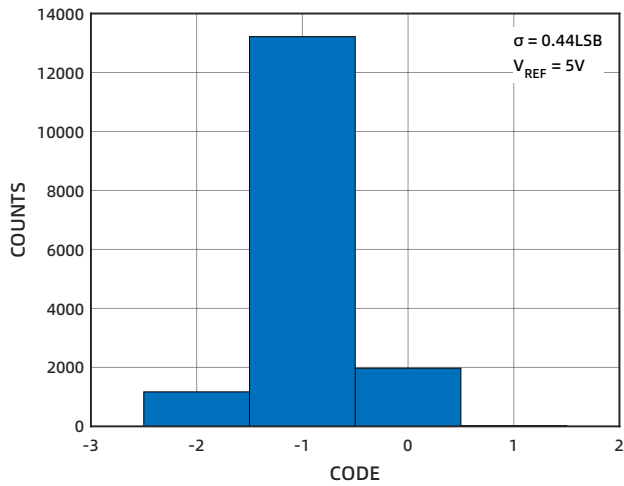
图 7 直流输入直方图（码中心，5V）
