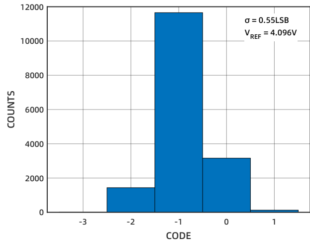
图 8 直流输入直方图（码中心，4.096V）
