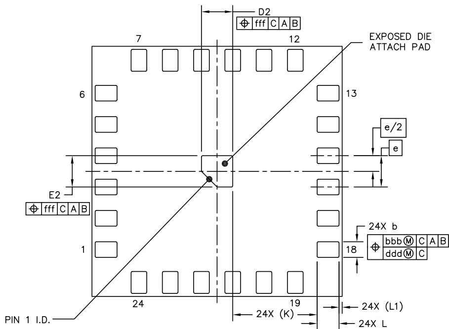
底视图
