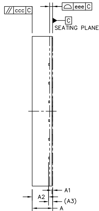
侧视图
