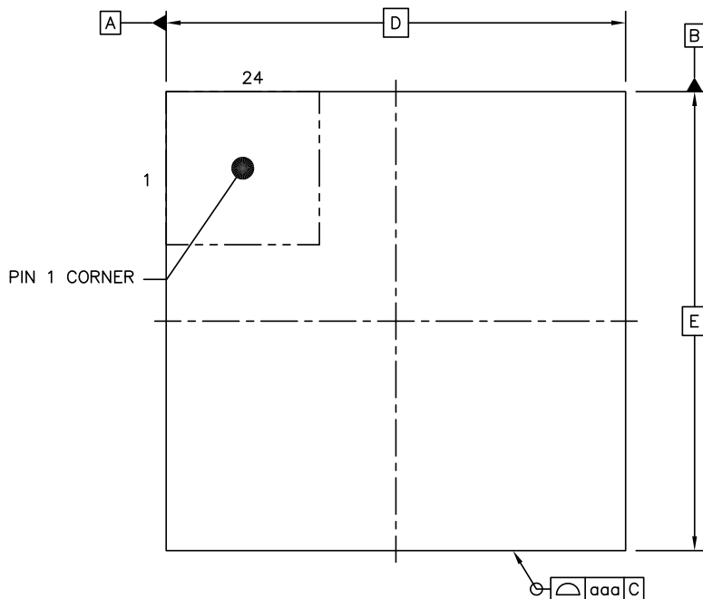
顶视图
