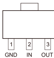
SOT89-3
