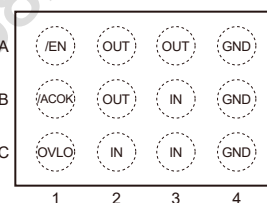
WLCSP-12L
