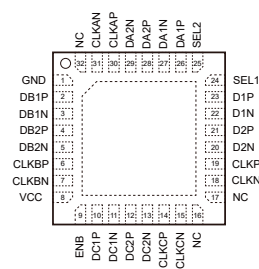
QFN4x4-32L
