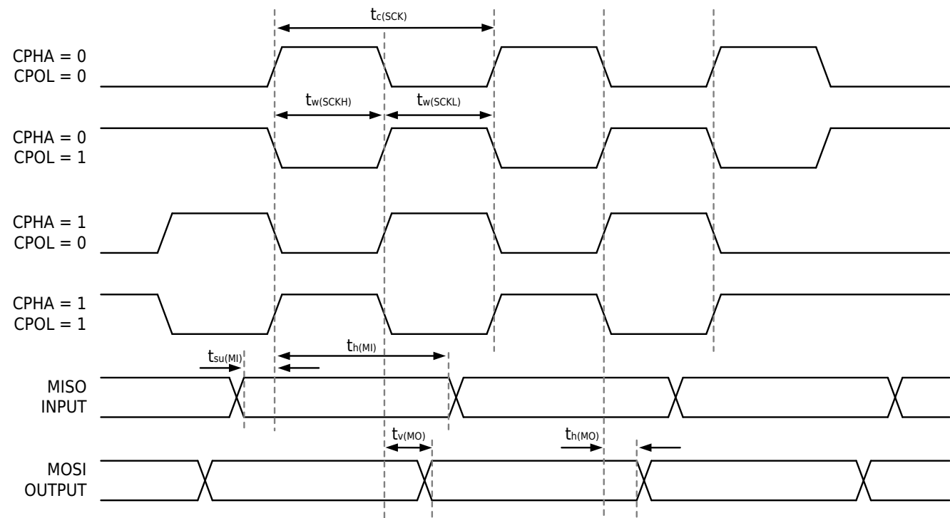
图 5-10 SPI 时序图（主机模式）
