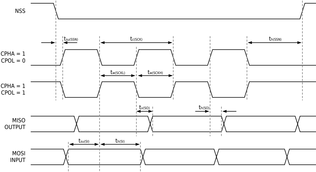
图 5-12 SPI 时序图（从机模式 CPHA=1）
