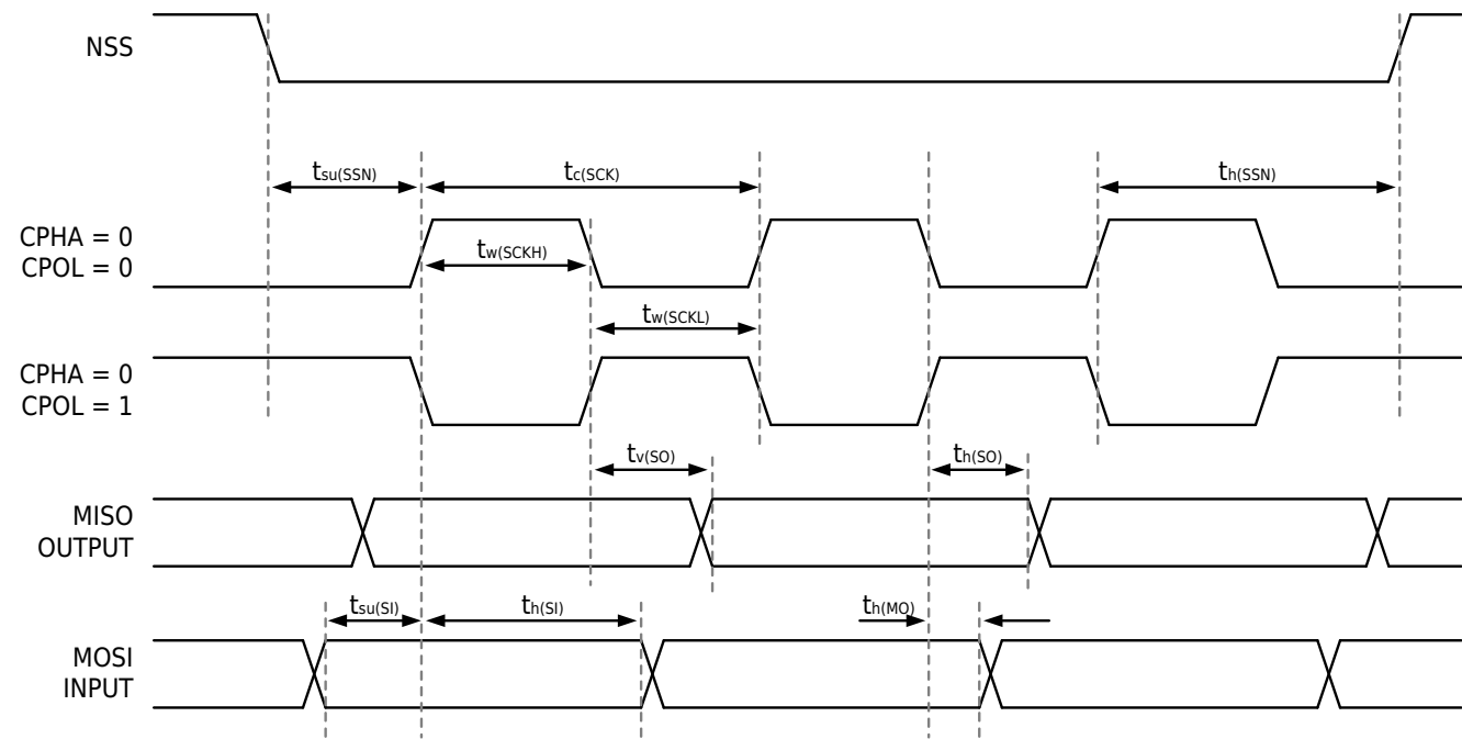
图 5-11 SPI 时序图（从机模式 CPHA=0）
