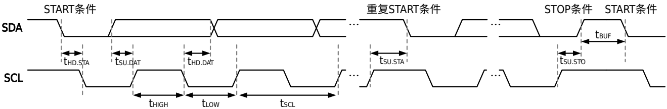
图 5-9 HSI2C/I2C 接口时序
