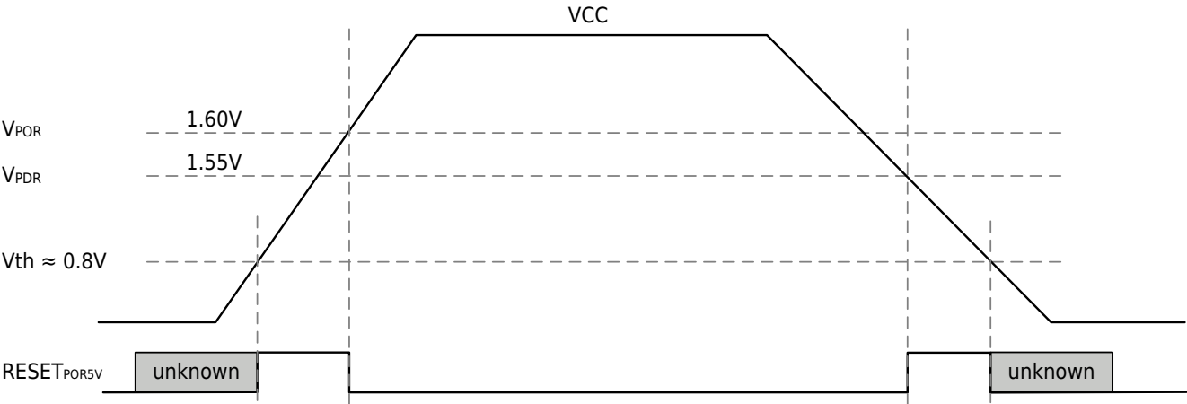
图 5-2 POR/PDR 示意图
