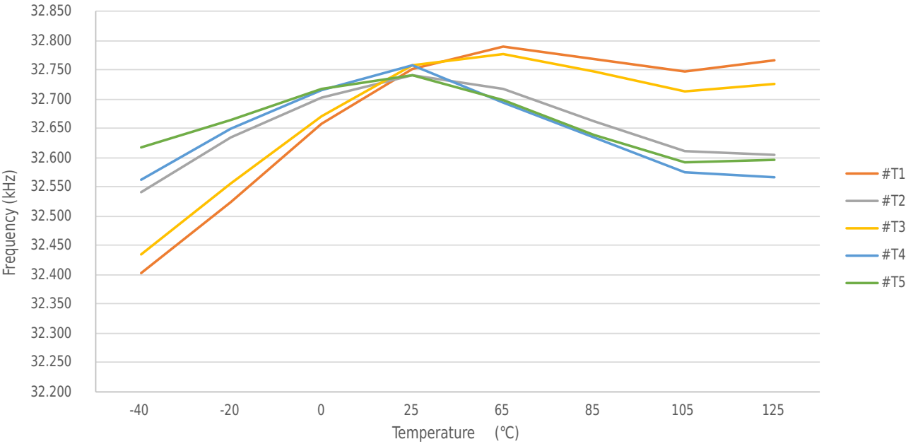
图 5-6 RCL 时钟频率变化曲线 (F CLK =32.768kHz, V CC =3.3V)
