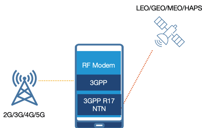
图: NTN网络主要构成示意图 (地面基站+NTN终端+卫星及高空平台)
