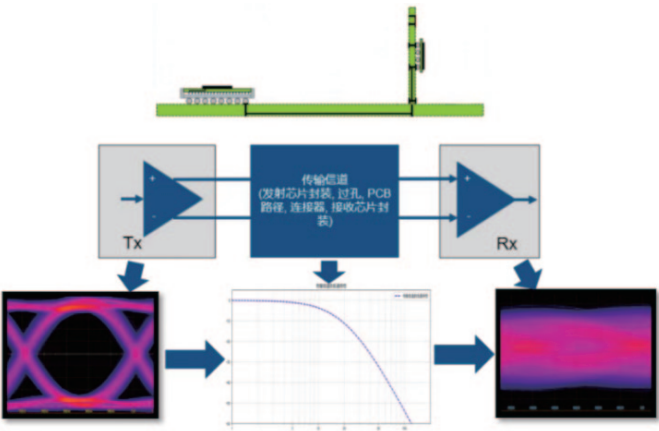
高速数字信号传输过程示意图
