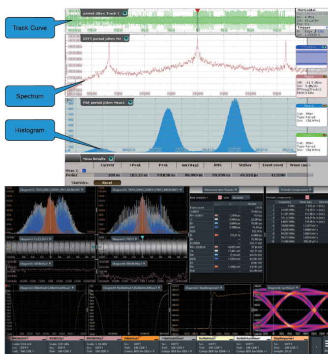
使用K12和K133/K134抖动分析选件测试TIE抖动及高级抖动/噪声分析
