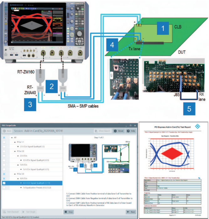
PCIE总线一致性测试示意图及测试软件界面
