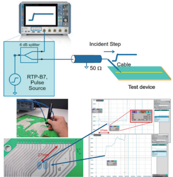
使用RTx示波器的TDR功能检测PCB电路板
