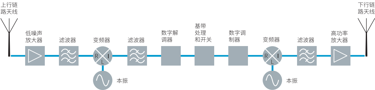
星载荷射频架构示意图
