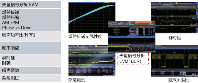
卫星载荷组件测试项与界面举例
