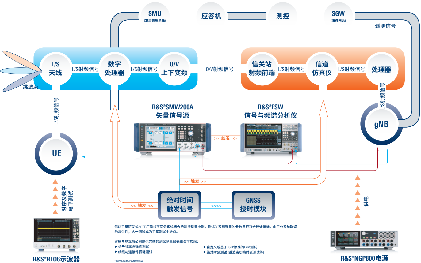
NTN 低轨卫星电测仪表连接逻辑图
