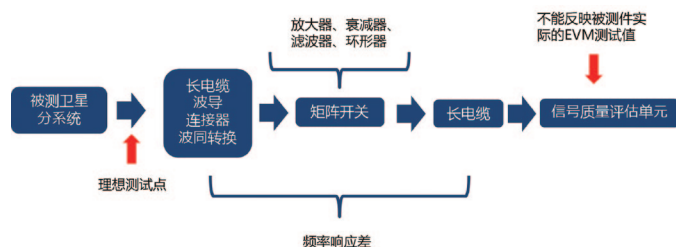
卫星AIT中的典型连图与测试点示意
