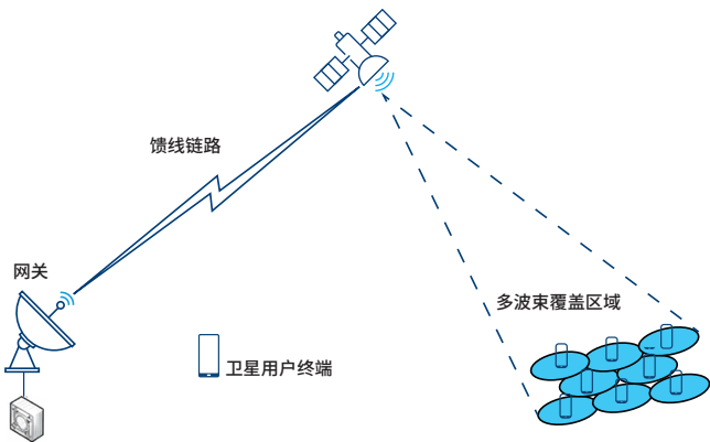
图3：多波束LEO卫星
