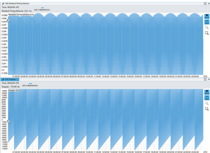
图9：时延和多普勒频移
