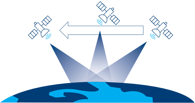
图2：准地球静止
