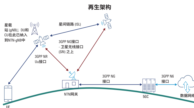
图2：NTN卫星网络架构
