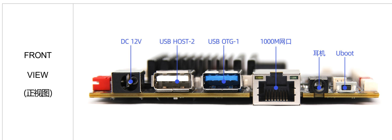
正视图:
