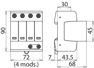
VT1 M TNS 385 CN 尺寸图
