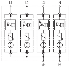
VT1 M TNS 385 CN 基本线路图
