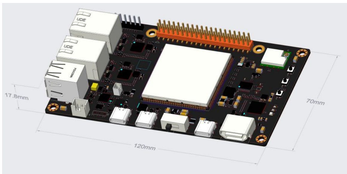
图 5-4 MYD-YT153-MINI 机械尺寸图 (单位: mm)
