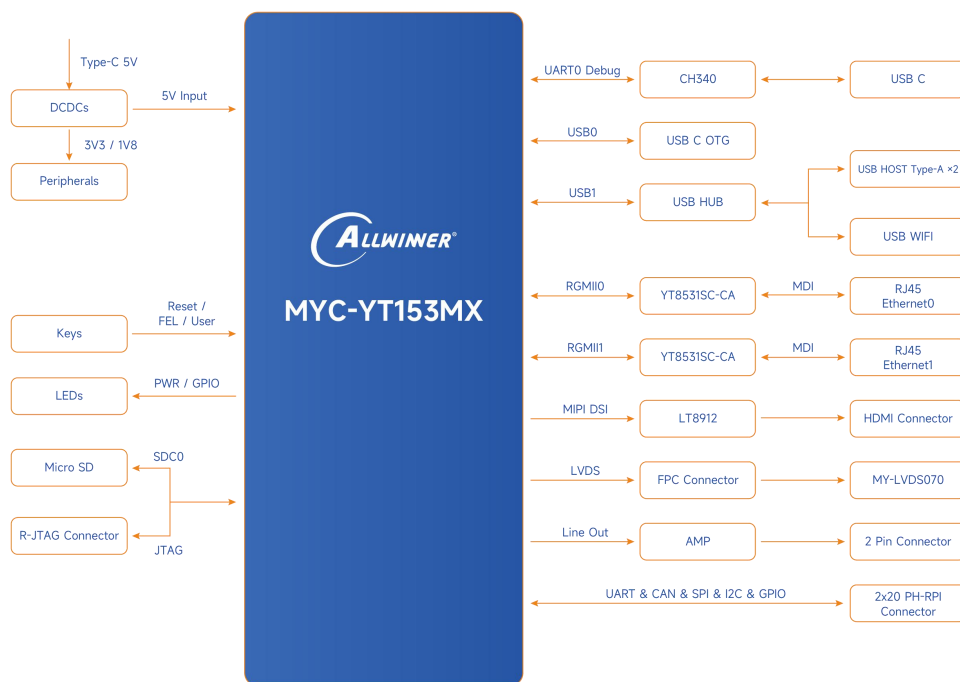
图 5-3 MYD-YT153MX-MINI 开发板系统框架图
