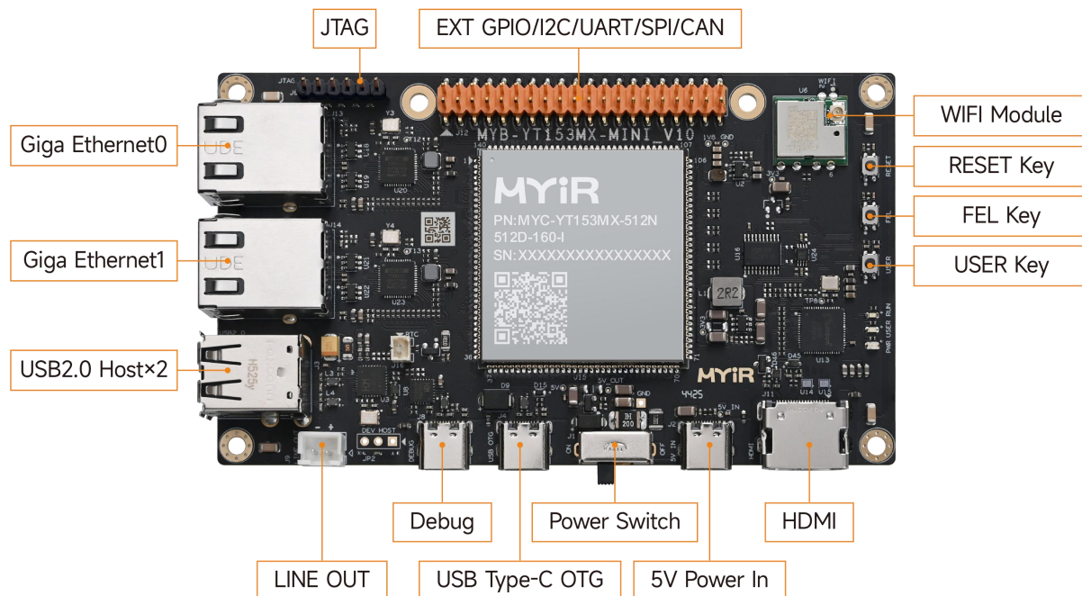
图 5-1 MYD-YT153MX-MINI 开发板正面接口标注图
