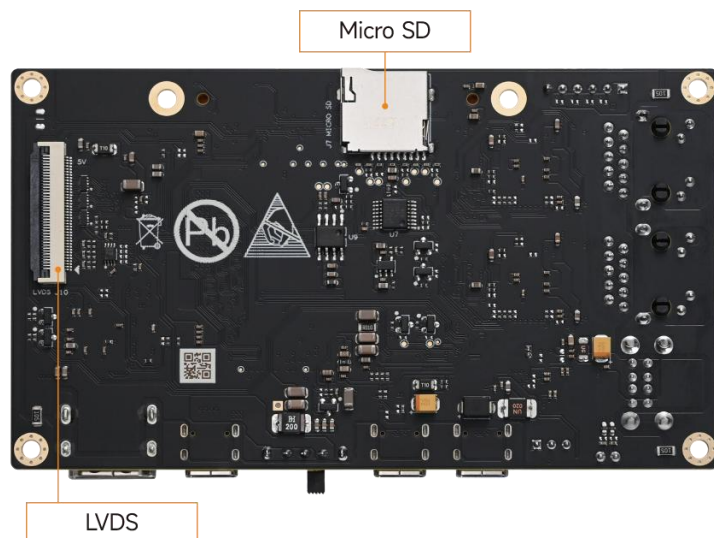
图 5-2 MYD-YT153MX-MINI 开发板背面接口标注图
