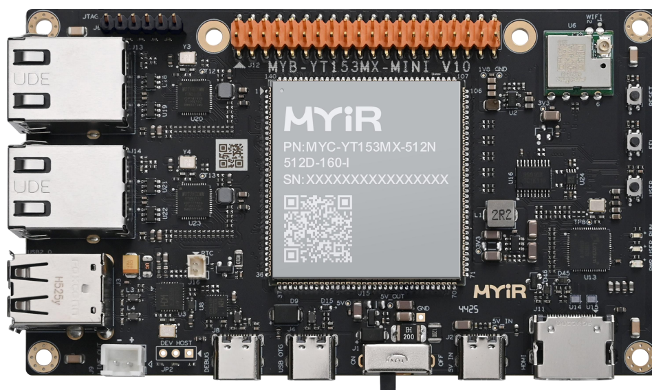
图 1-1 MYD-YT153MX-MINI 开发板
