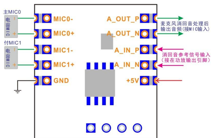
双电容麦克风连接图
