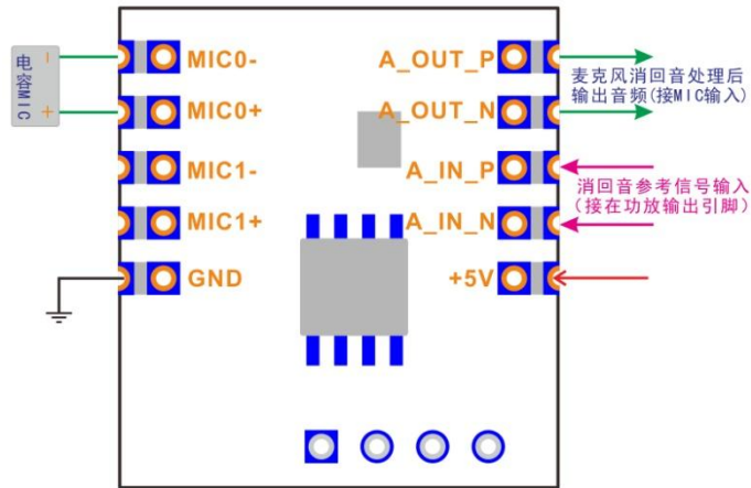
单麦克风应用连接图
