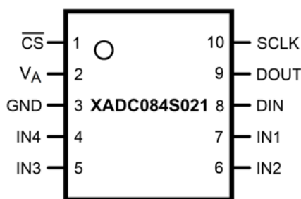
引脚图
