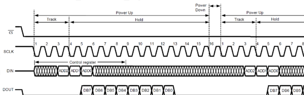
XADC084S021 操作时序图
