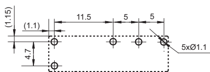
安装孔尺寸 (底视图)
