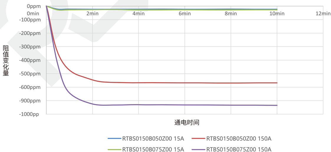
RTBS0150系列分流器通电电阻值变化情况
