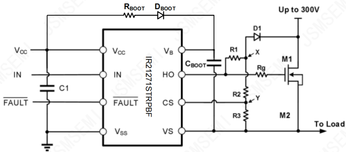
图 7-2 典型应用电路图
