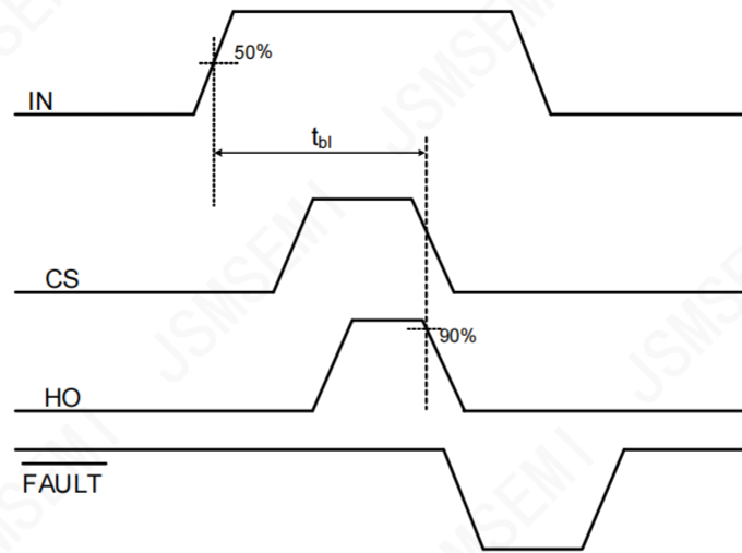
图 6-3 消隐时间定义
