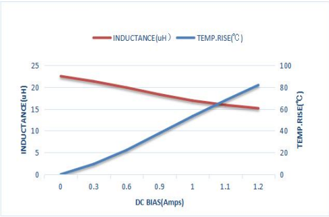
ZETC252010S220MBT-LF
