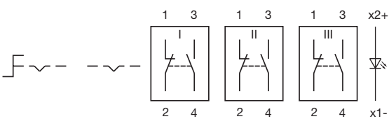
Wiring diagram 279
