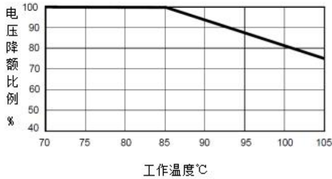
额定电压降额曲线
