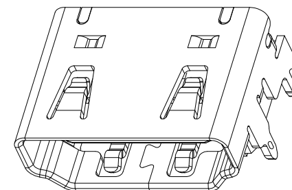
脚有凸点
