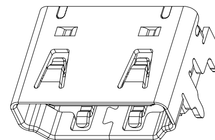
脚无凸点
