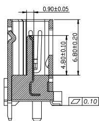
SECTION-A
