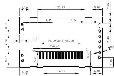
背视图
