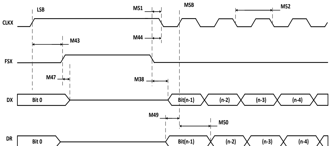
图 6-30 McBSP 作为 SPI 主、从模式时序 : CLKSTP=10b , CLKXP=1
