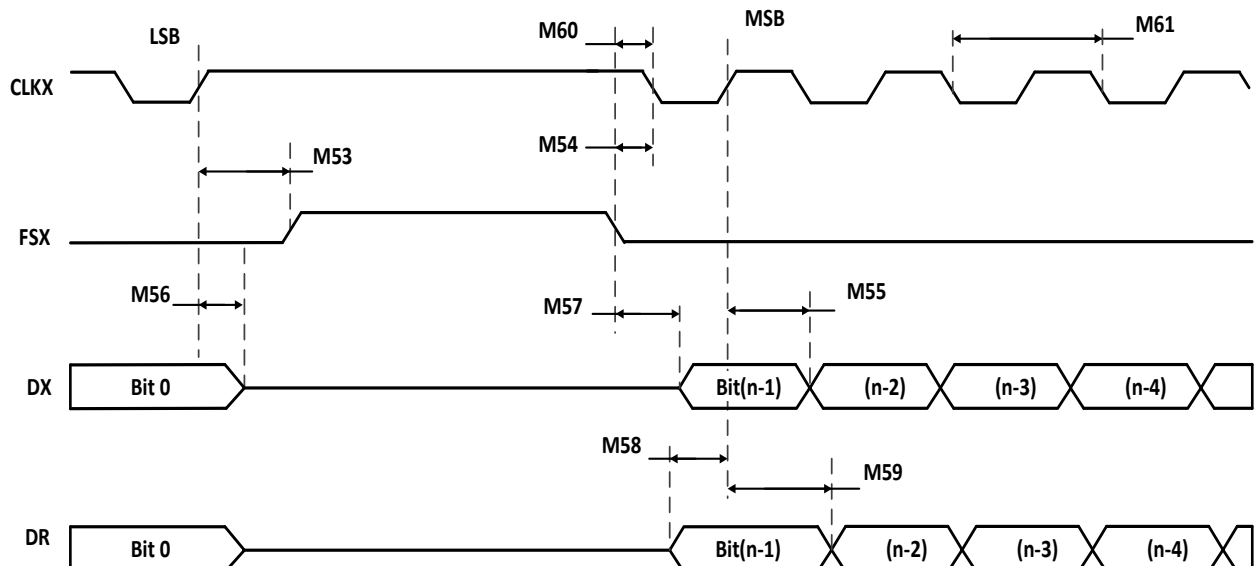
图 6-31 McBSP 作为 SPI 主、从模式时序 : CLKSTP=11b, CLKXP=1
