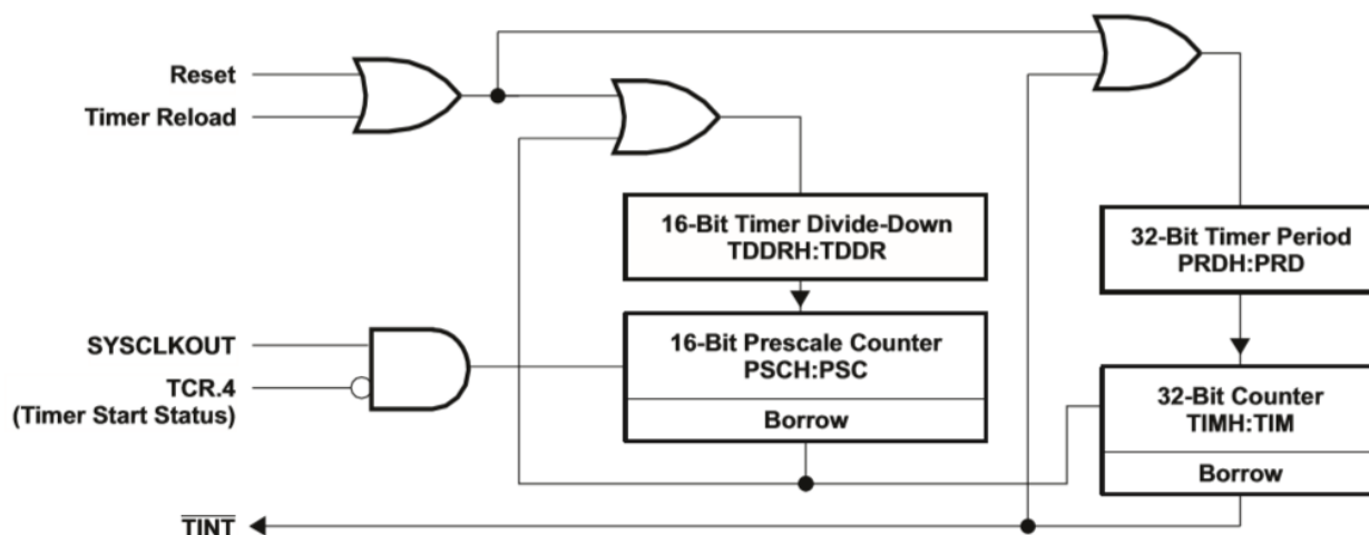
图 4-2 CPU 定时器
