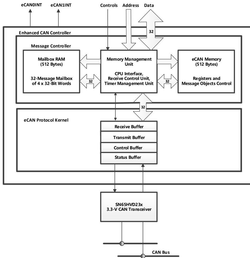
图 4-12 eCAN 功能框图和接口电路
