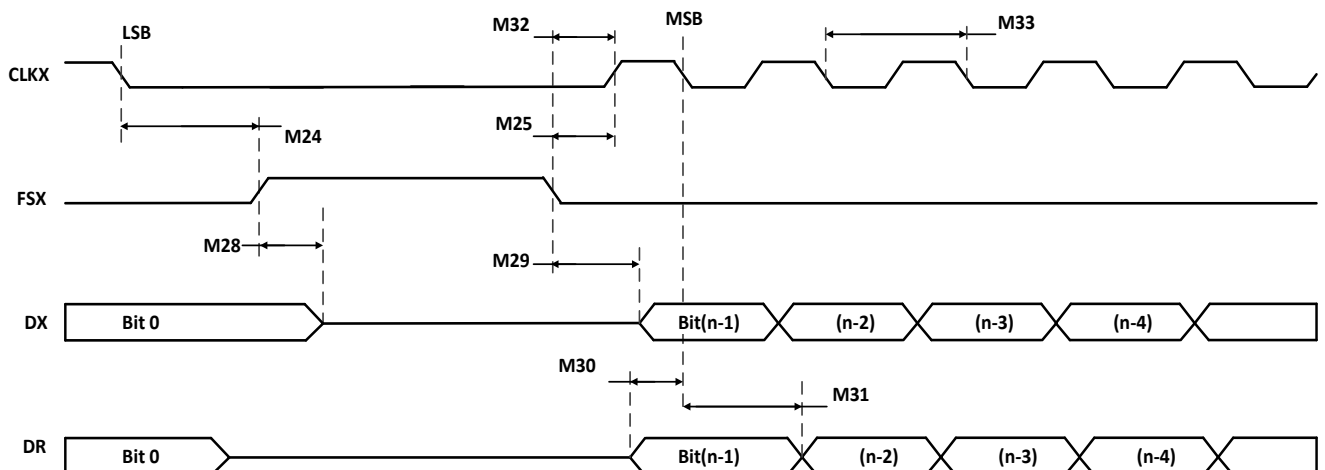
图 6-28 McBSP 作为 SPI 主、从模式时序 : CLKSTP=10b, CLKXP=0
