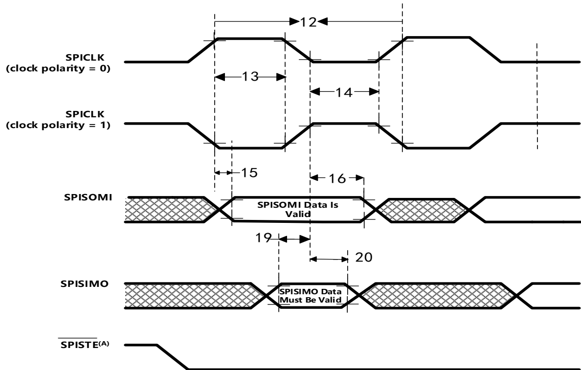
图 6-20 SPI 从模式外部时序 ( 时钟相位 = 0 )
