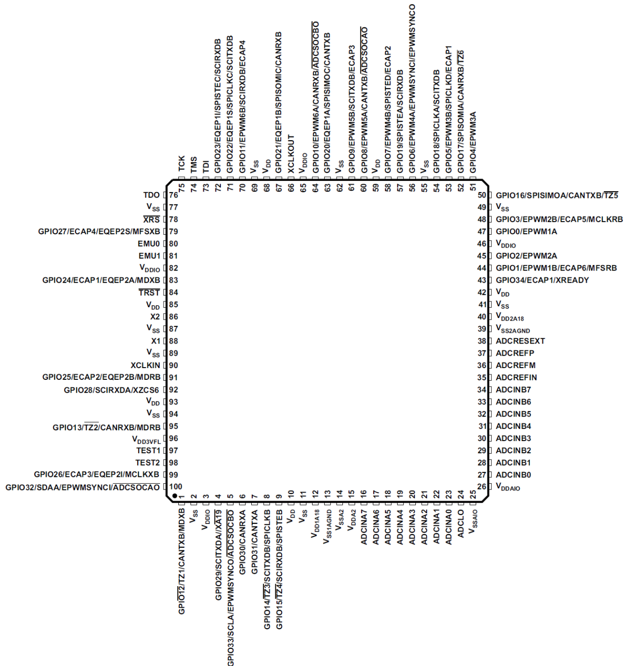
图 2-1 AVP32F08 100 引脚 QP（LQFP 顶视图）
