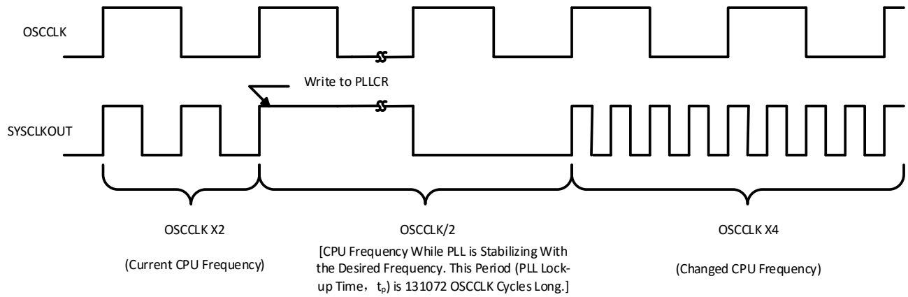
图 6-8 写入 PLLCR 寄存器过程时序示例
