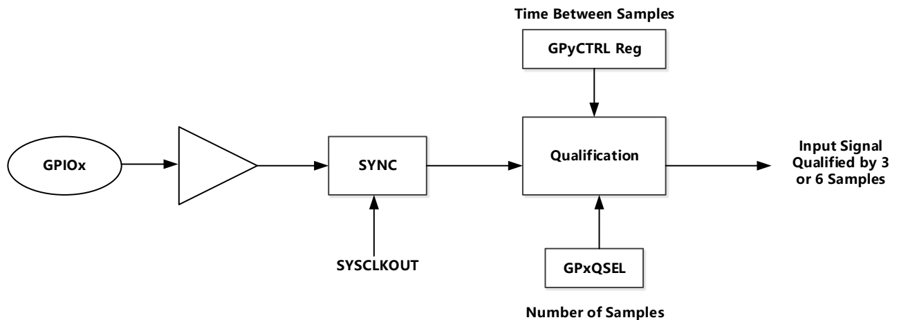
图 4-19 采样窗口的限定
