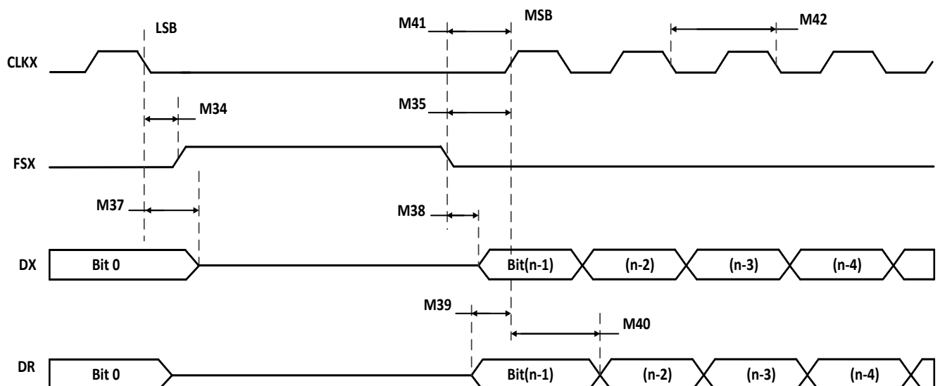
图 6-29 McBSP 作为 SPI 主、从模式时序: CLKSTP=11b, CLKXP=0
