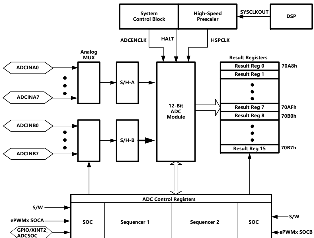
图 4-8 ADC 模块的功能框图
