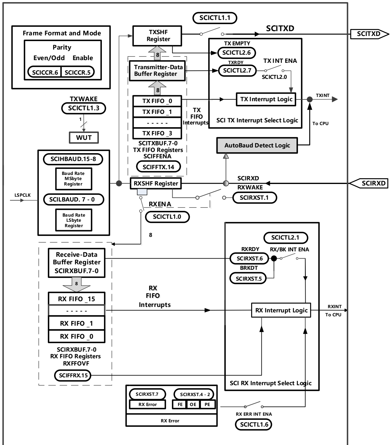
图4-15 显示了SCI 模块功能框图。
