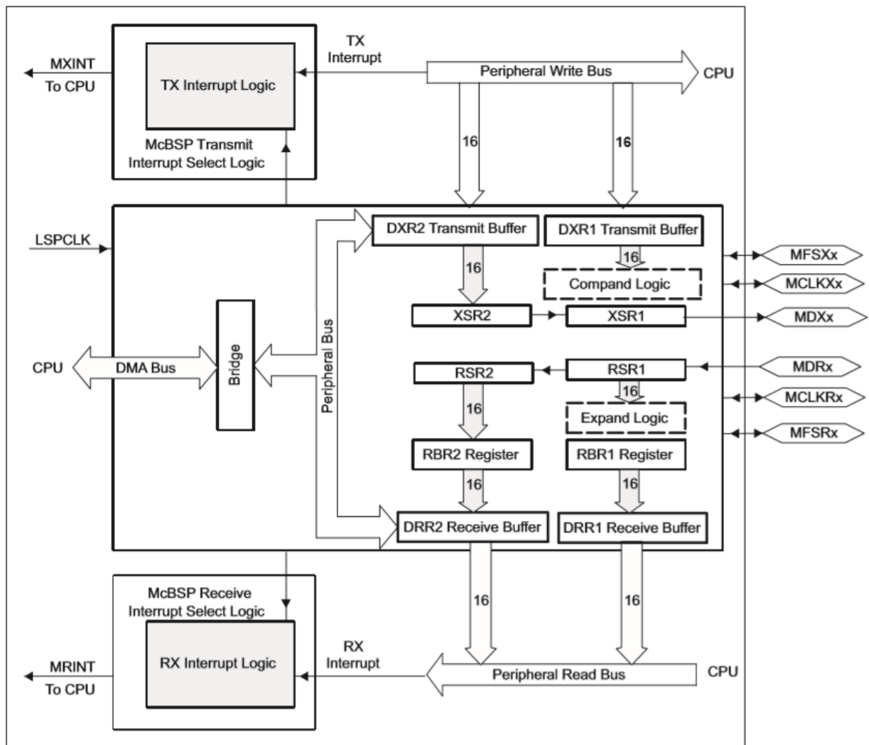
图 4-11 McBSP 模块的功能框图。
