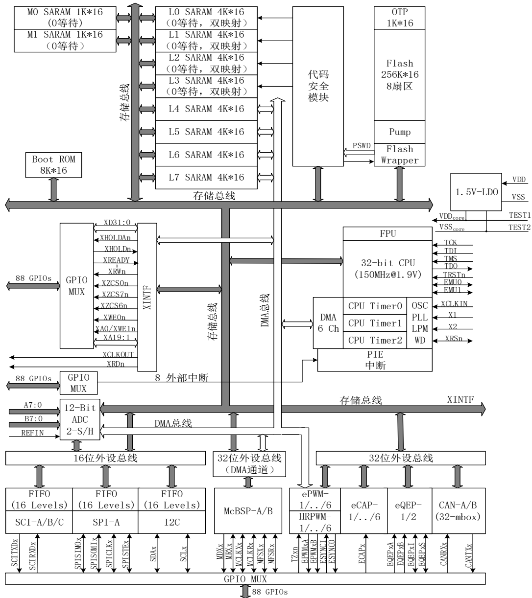
图 3-1 功能框图
