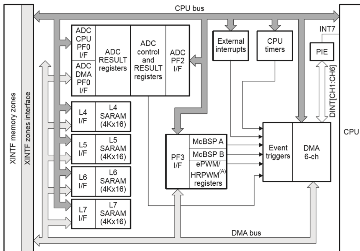
图 4-1 DMA 功能功能框图
