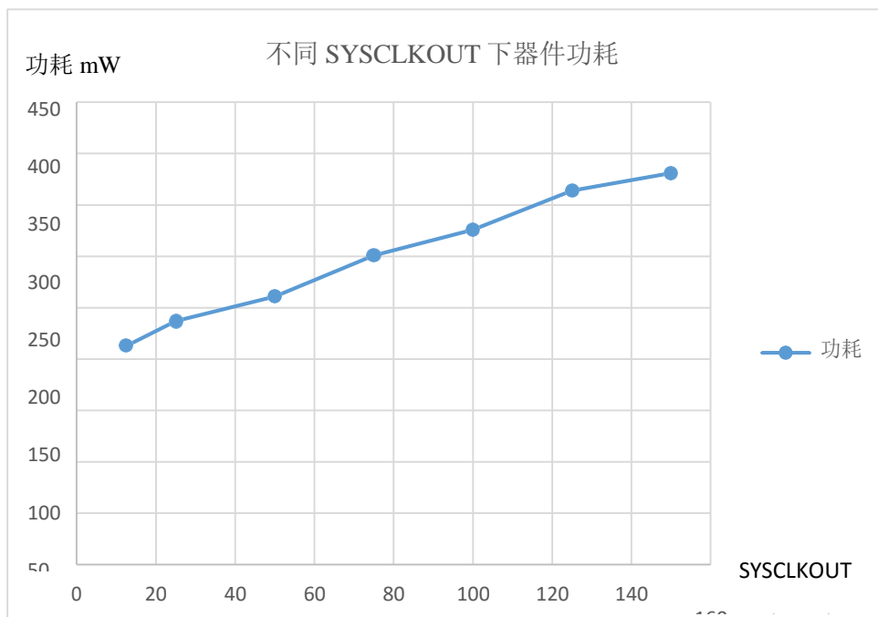
图 6-2 典型运行功率与频率间的关系
