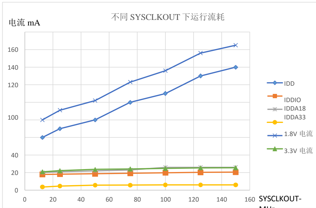
图 6-1 典型运行电流与频率间的关系
