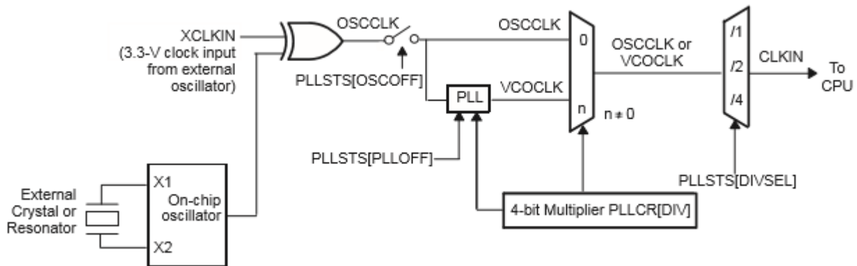
图 3-7 OSC 和 PLL 模块功能框图
