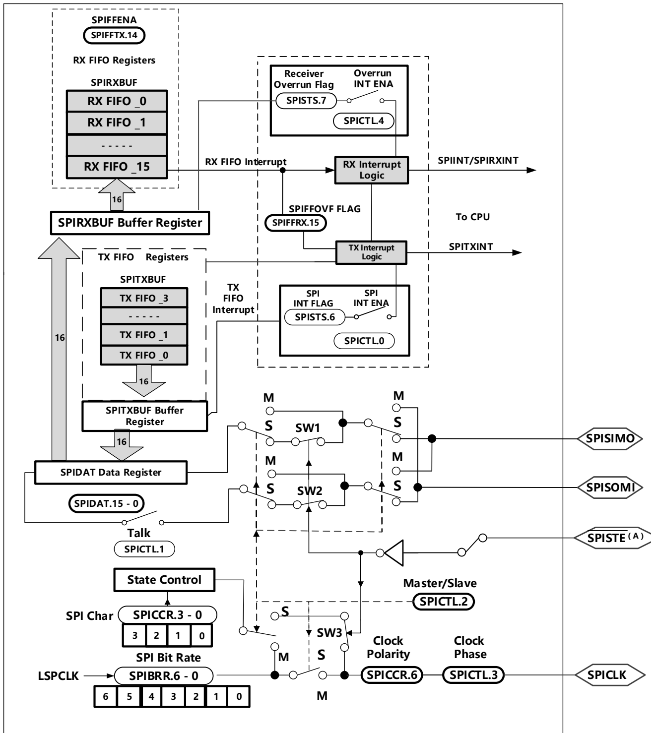
图 4-16 SPI 模块功能框图（受控模式）
