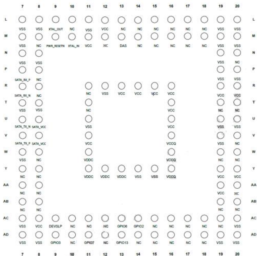
图 3-2 uSIC 主控引脚分配
