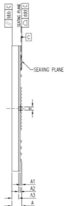
侧视图
