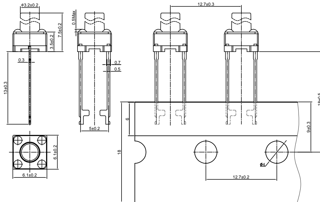
P.C.B. LAYOUT
