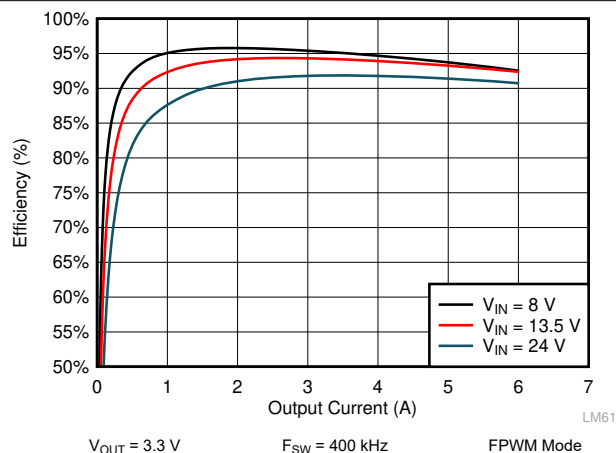
图 10-6. LM61460-Q1 Efficiency
