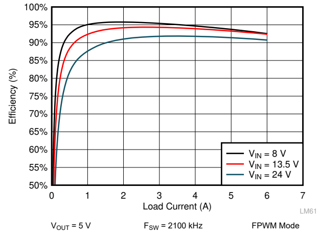
图 10-12. LM61460-Q1 Efficiency
