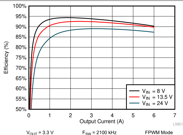
图 10-8. LM61460-Q1 Efficiency
