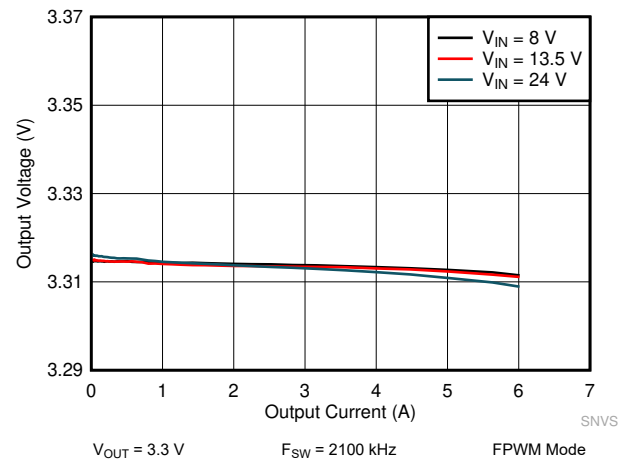
图 10-16. LM61460-Q1 Load and Line Regulation
