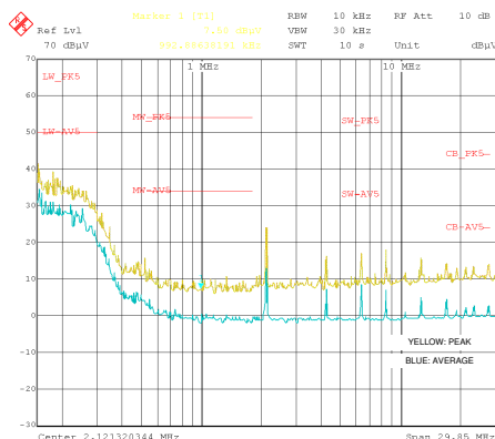
传导 EMI: V_{OUT} = 5V , I_{OUT} = 5A
