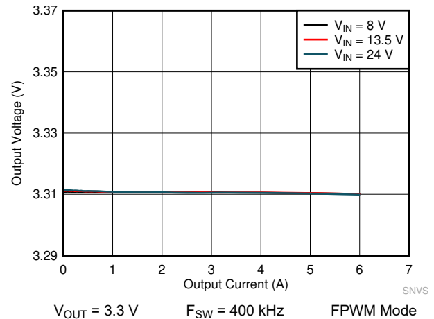
图 10-14. LM61460-Q1 Load and Line Regulation
