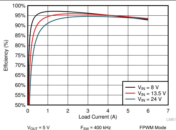
图 10-10. LM61460-Q1 Efficiency
