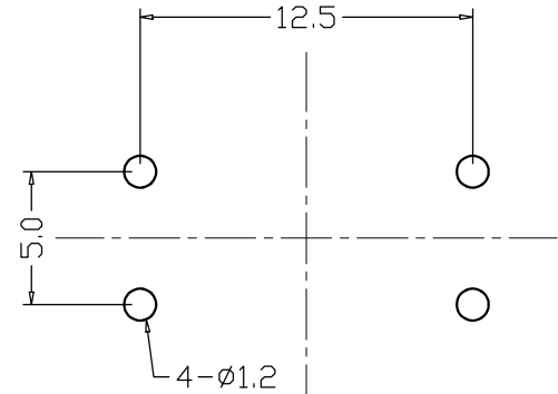
PCB线路板图
