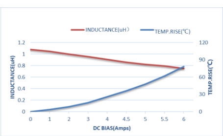
ZETC252012S1R0MBT-LF
