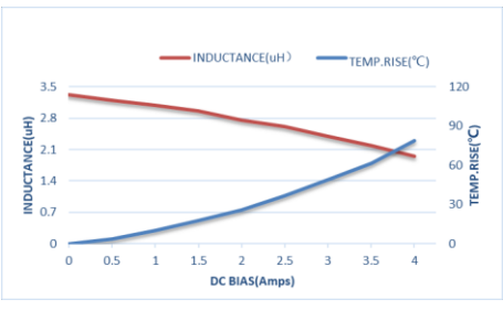
ZETC252012S3R3MBT-LF
