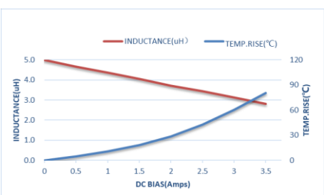
ZETC252012S4R7MBT-LF
