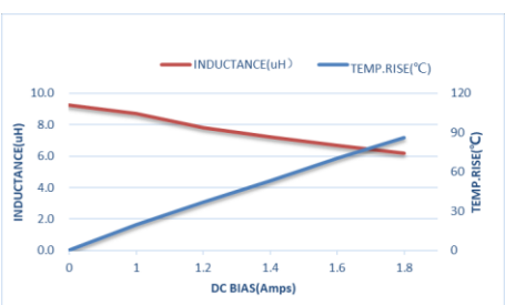
ZETC252012S100MBT-LF
