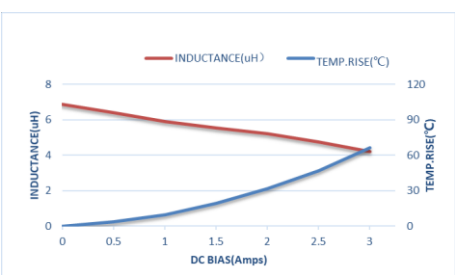
ZETC252012S6R8MBT-LF
