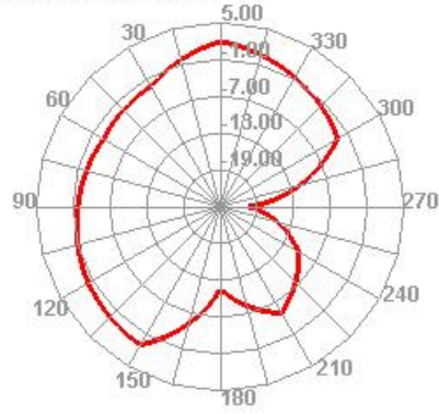
2400.000MHz E2
