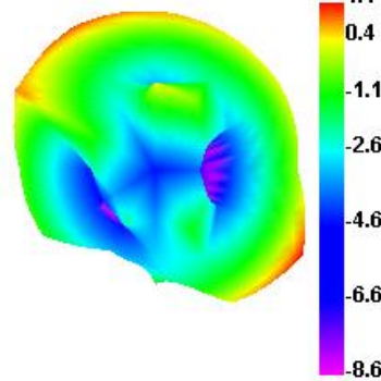
5160.000MHz E1
