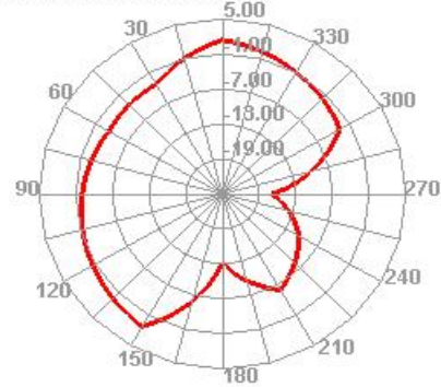
2410.000MHz H
