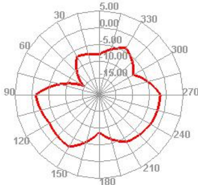
5160.000MHz E1
