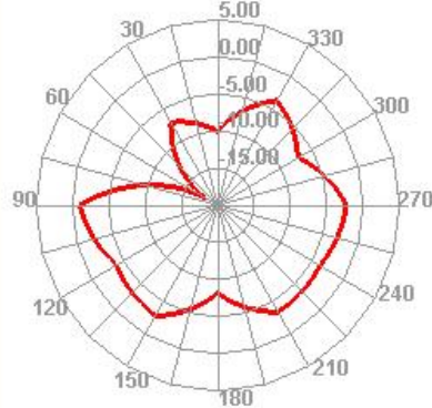
5160.000MHz
