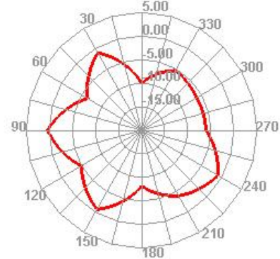
5160.000MHz H
