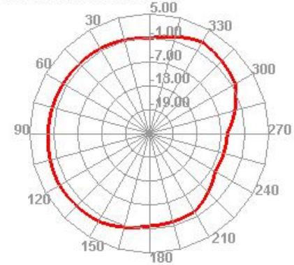
5160.000MHz E2
