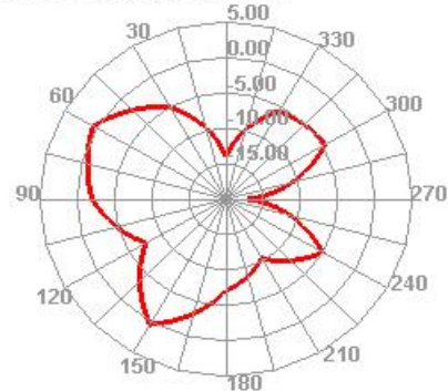
2410.000MHz E2
