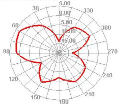
2410.000MHz E1
