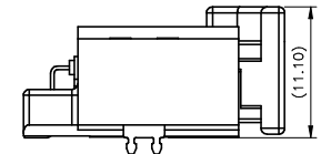
16~20 PIN
