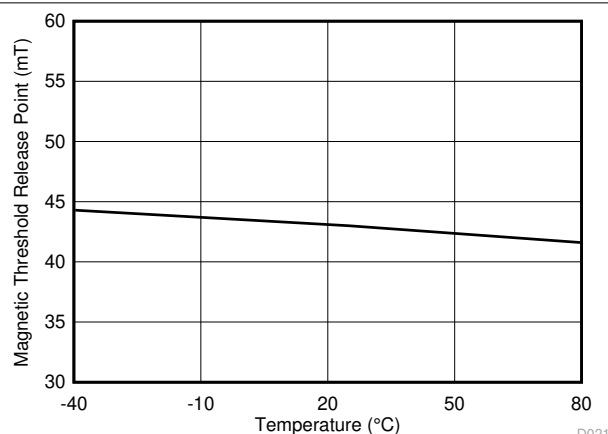
图 6-9. ZE 版本 |B_{RP}| 与温度间的关系
