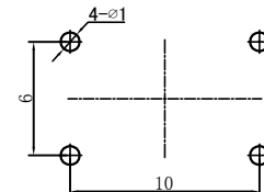
P. C. B. LAYOUT
