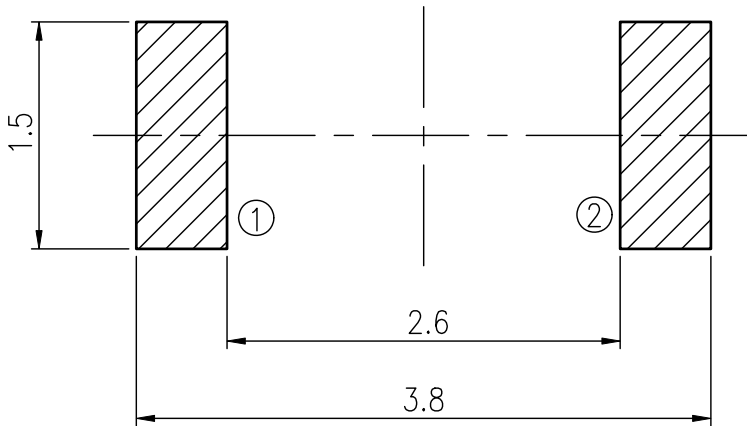
P.C.B. LAYOUT
