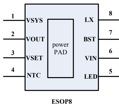
图 2 IP2325_3S 引脚图
