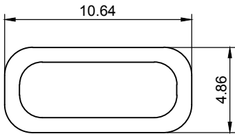
防水圈尺寸
