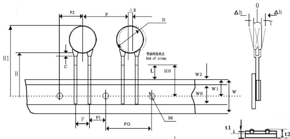
▼ 10.1-4: 孔距 12.7mm/单内弯型/脚距 P=5.0mm
