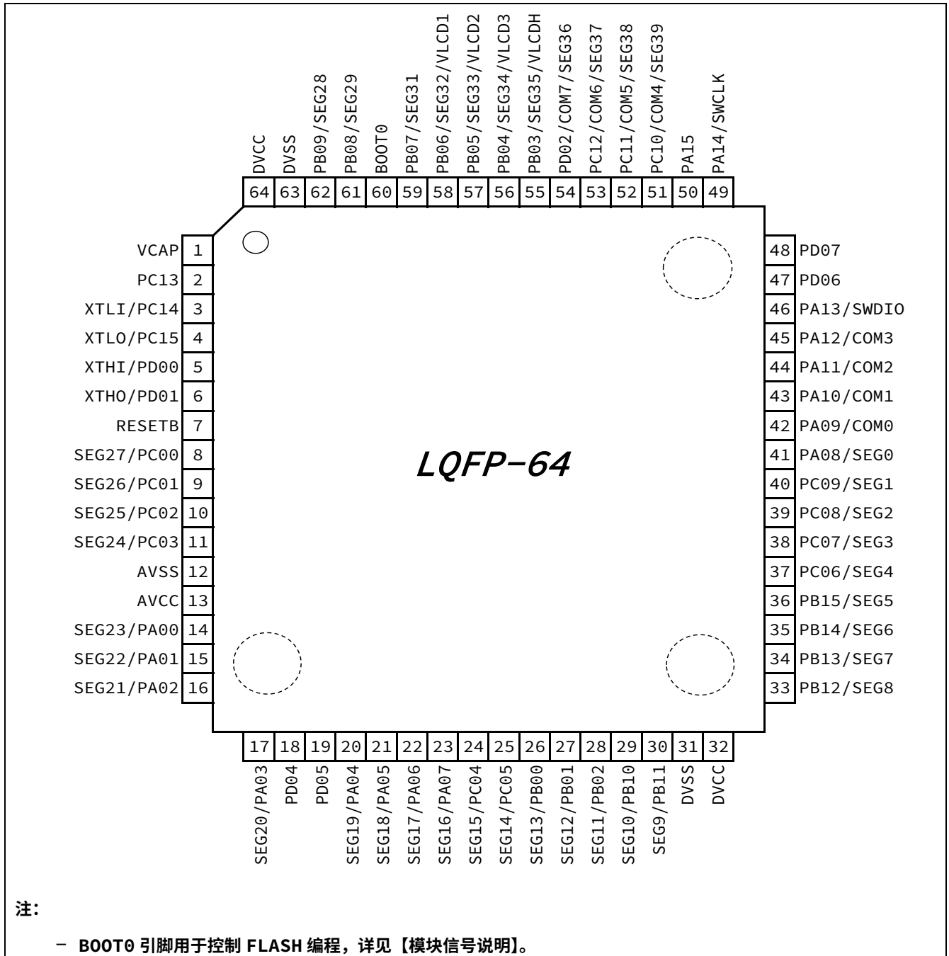
HC32L136K8TA
