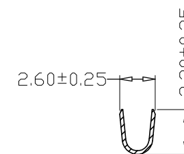
SEC:B-B
